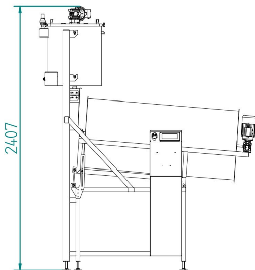
VISTA LATERAL
