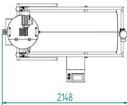
VISTA PLANTA
